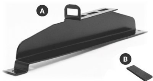
A - Uchwyt do panelu fotowoltaicznego B - Uszczelka (2szt./mocowanie)
